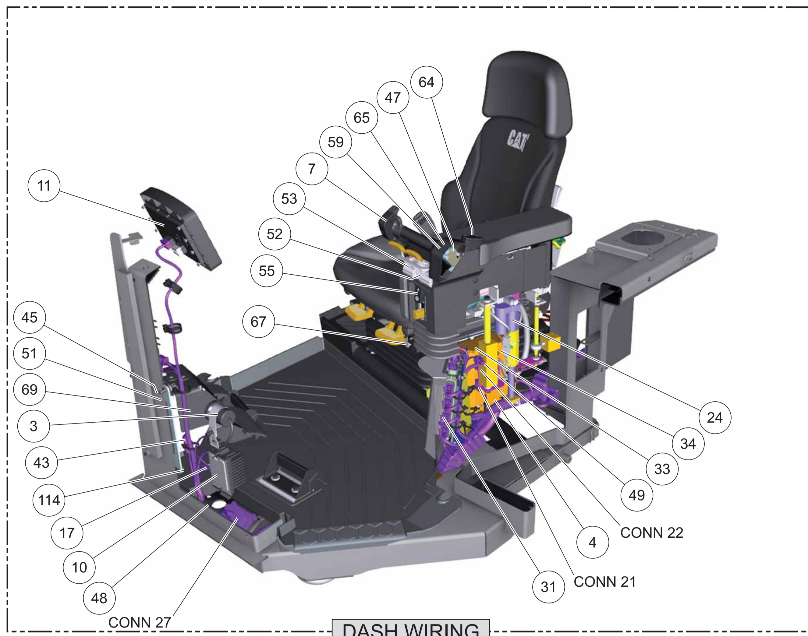
DASH WIRING
